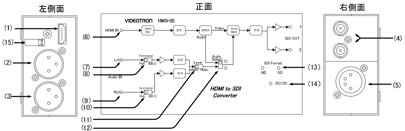
図B-1 各部の名称と働き
