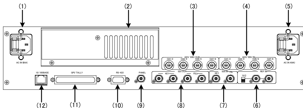
図3-2 本体背面
