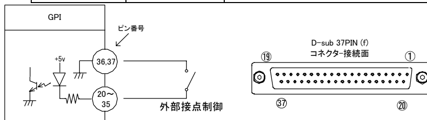
図6-1 GPI仕様
