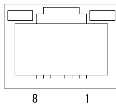
図6-4 10/100BASEコネクター
