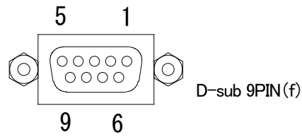
図6-3 RS-422コネクター
