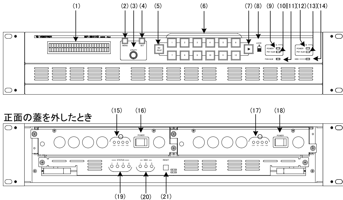
図3-1 本体正面
