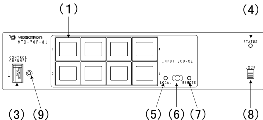
図 3.5 MTX-70P-81 正面図
