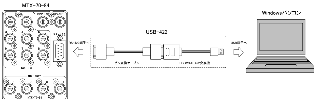
図 4.7a パソコンから RS-422 制御
