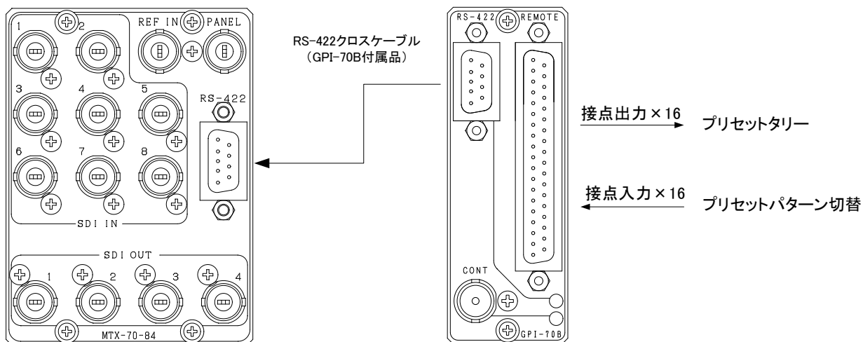
図 4.90 GPI-70B 接続図
