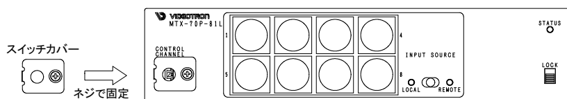
図 3.8 MTX-70P-81L スイッチカバー実装図
