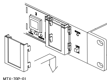
図4.121 MTX-70P-01の取り付け方
