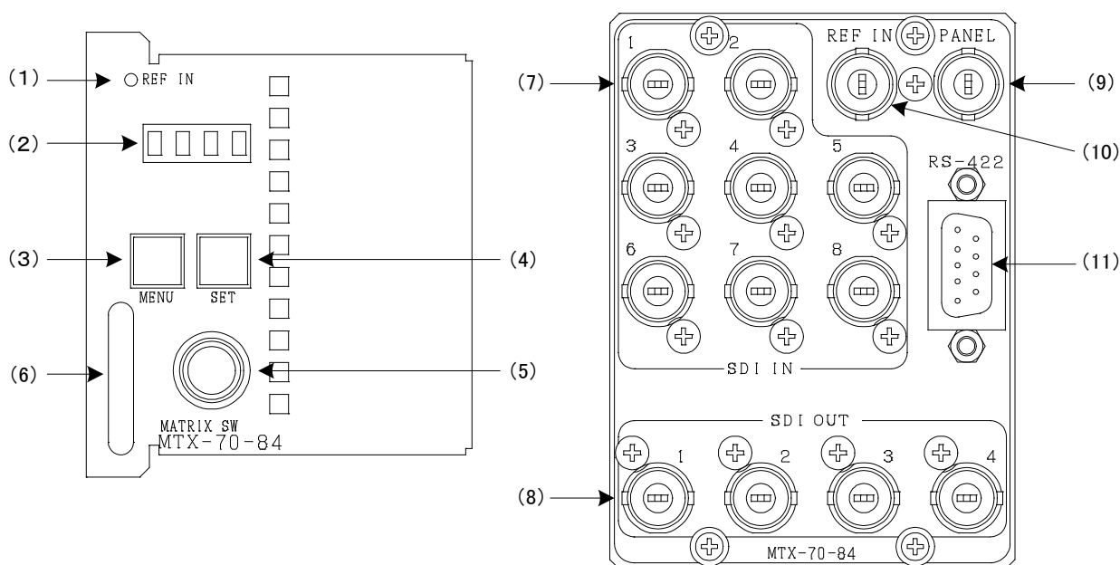
図 3.1 メインモジュール/コネクタモジュール正面図
