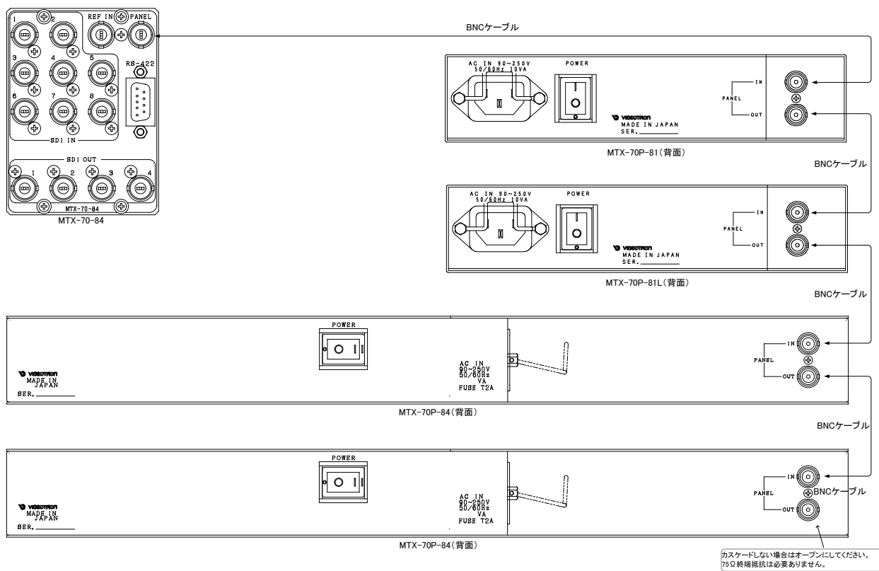
図4.122 カスケード接続例
