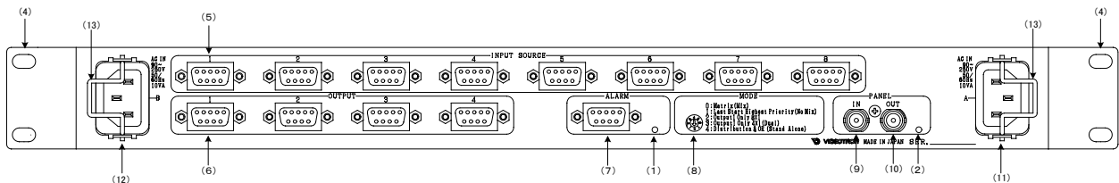
図 3.2 本体背面図
