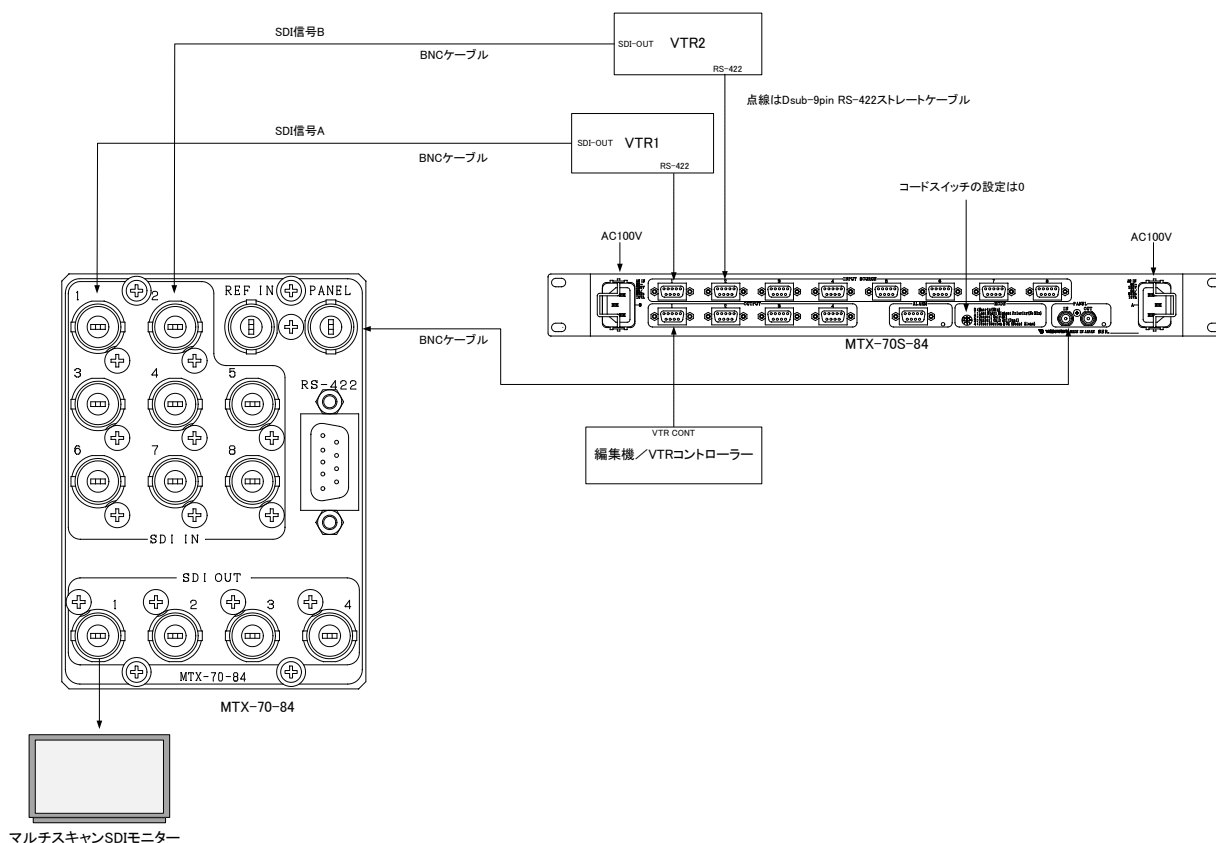
図 2.1 機能チェック接続図
