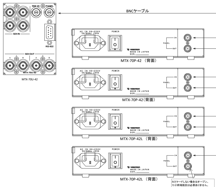
図 4.122 カスケード接続例
