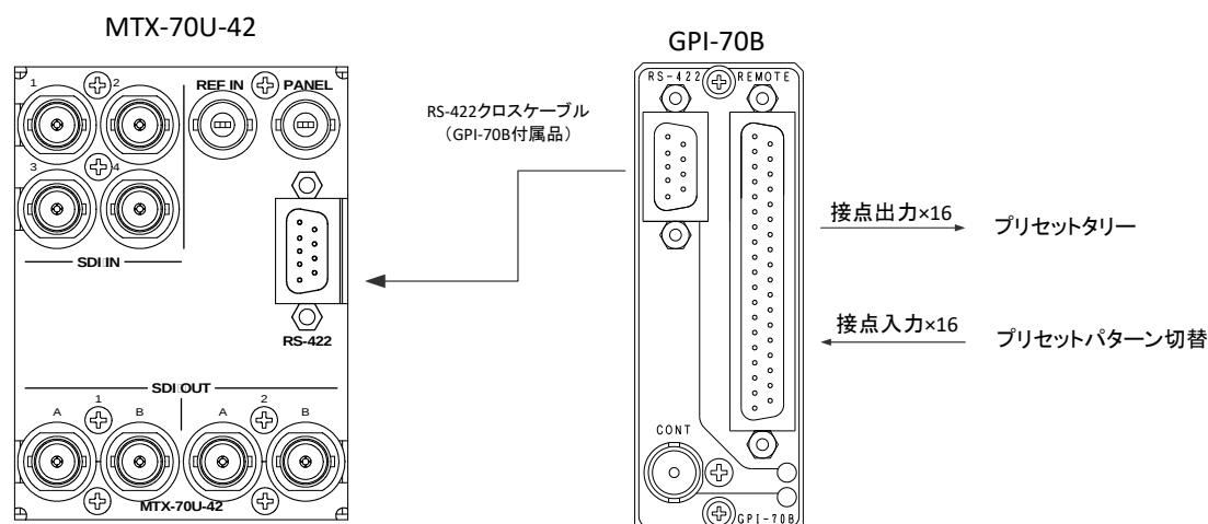
図 4.90 GPI-70B 接続図
