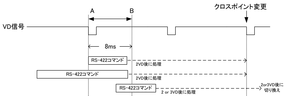
図 4.78 RS-422 制御タイミングチャート(DIPSW1=OFF)
