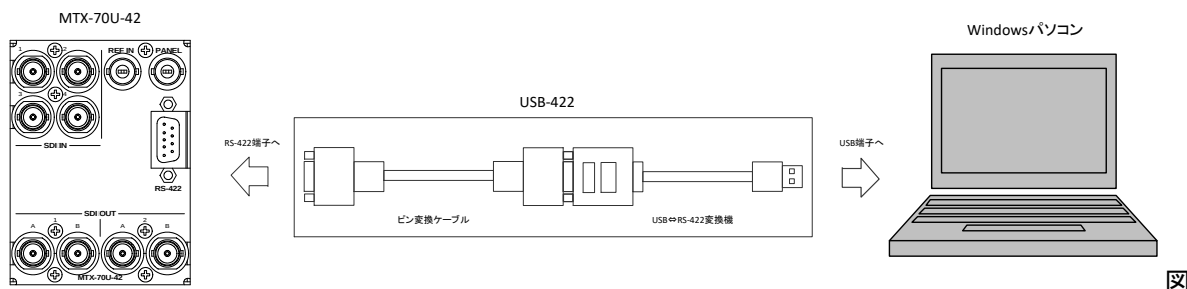
4.7a パソコンから RS-422 制御
