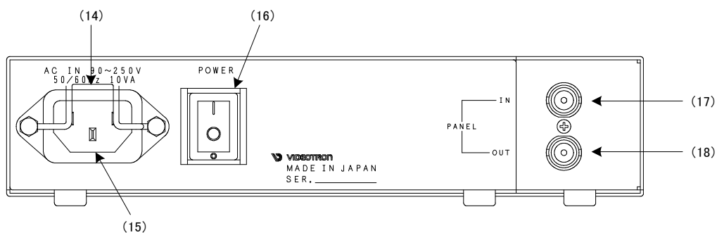
図 3.5 MTX-70P-42、MTX-70P-42L 背面図
