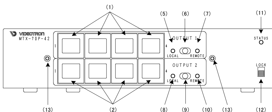
図 3.3 MTX-70P-42 正面図
