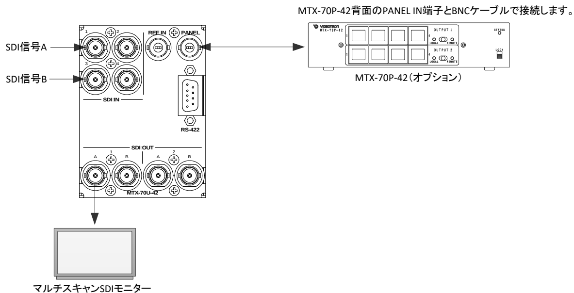
図 2.1 機能チェック接続図
