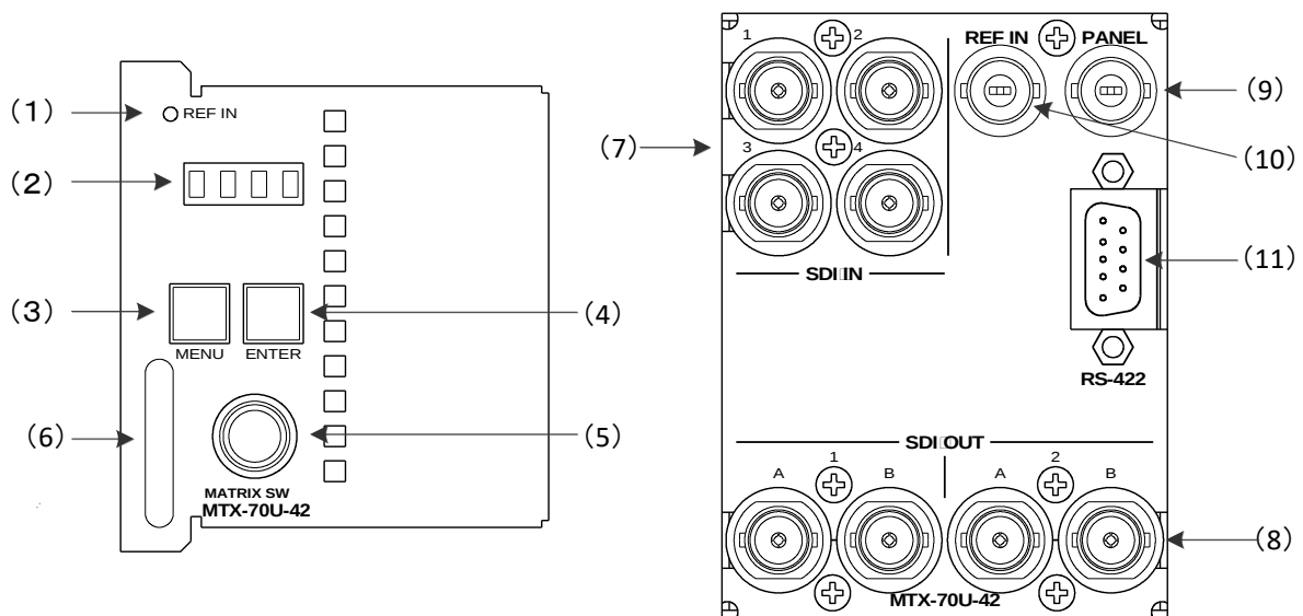
図 3.1 メインモジュール／コネクタモジュール正面図
