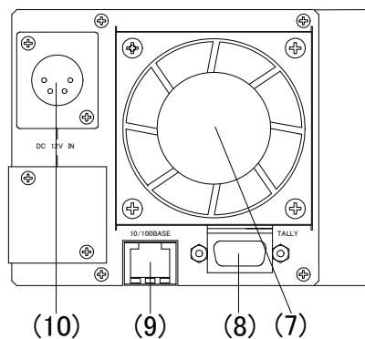
図 3-5 各部の名称(背面)
