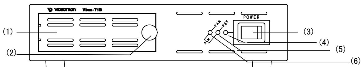
図 3-1 各部の名称(筐体正面)
