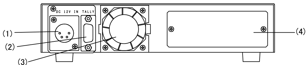
図 3-3 各部の名称(筐体背面)
