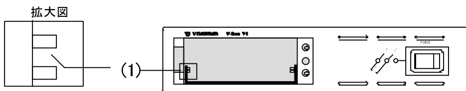
図 3-2 各部の名称(フロントパネルを取り外した状態)
