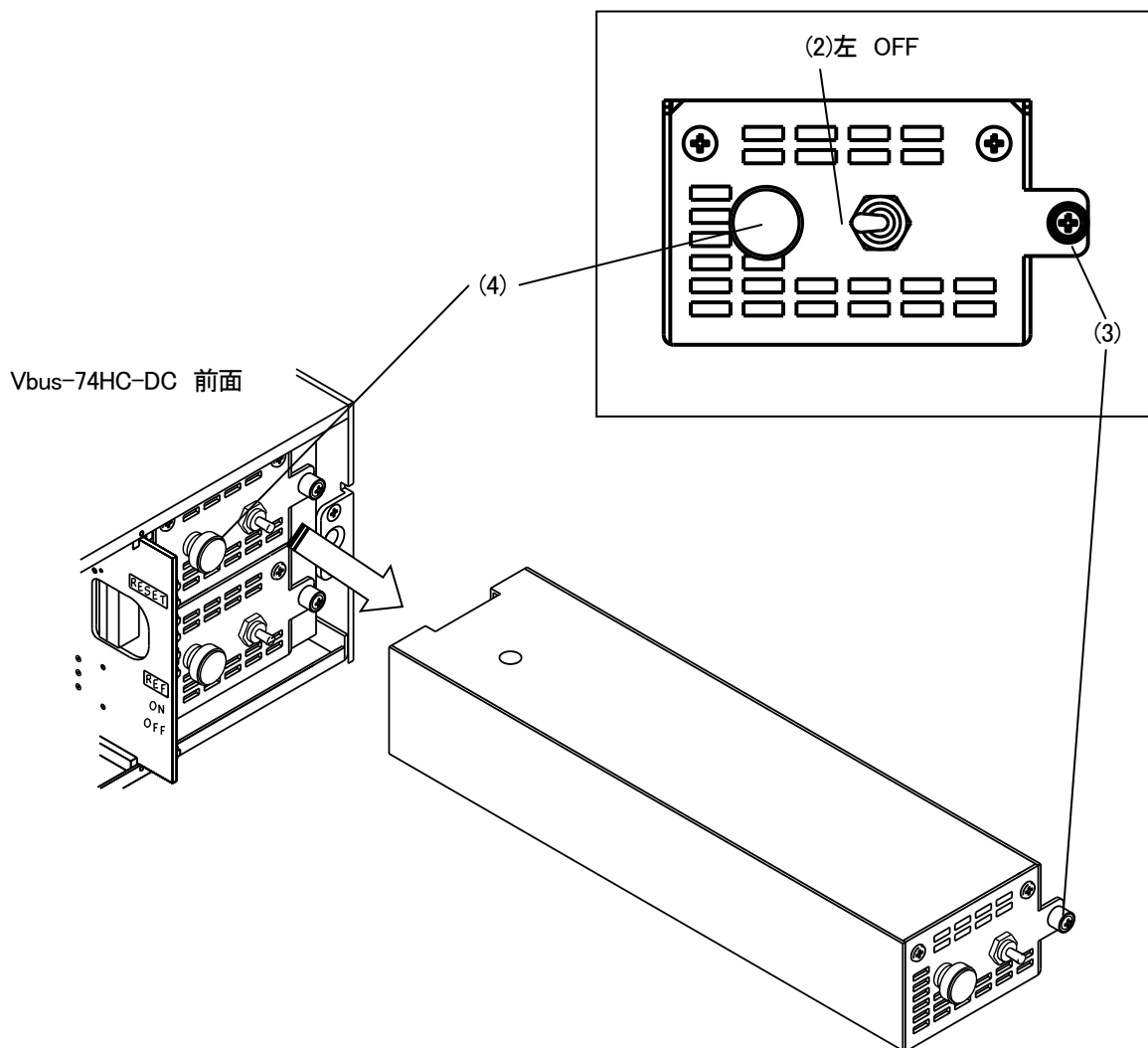
図 5-2 電源ユニット 取り外し方法
