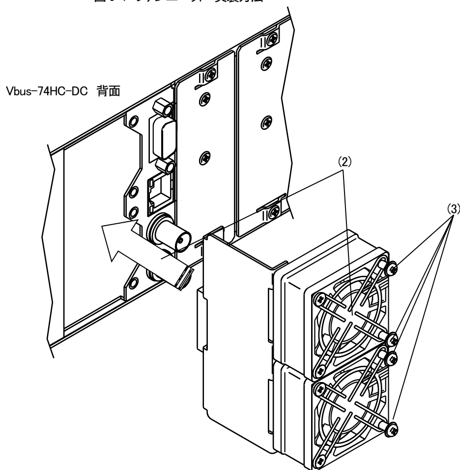
図 6-1 ファンユニット 実装方法
