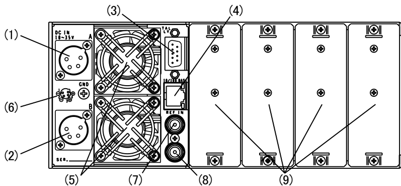
図 3-2 各部の名称(背面)
