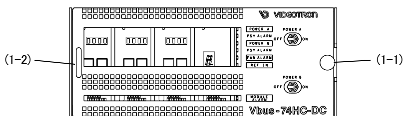
図 5-2 電源ユニット 取り外し方法
