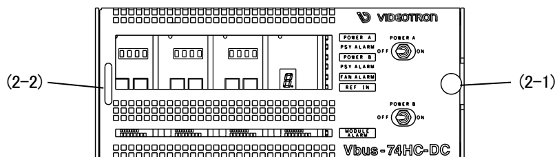
図 5-1 電源ユニット 増設方法
