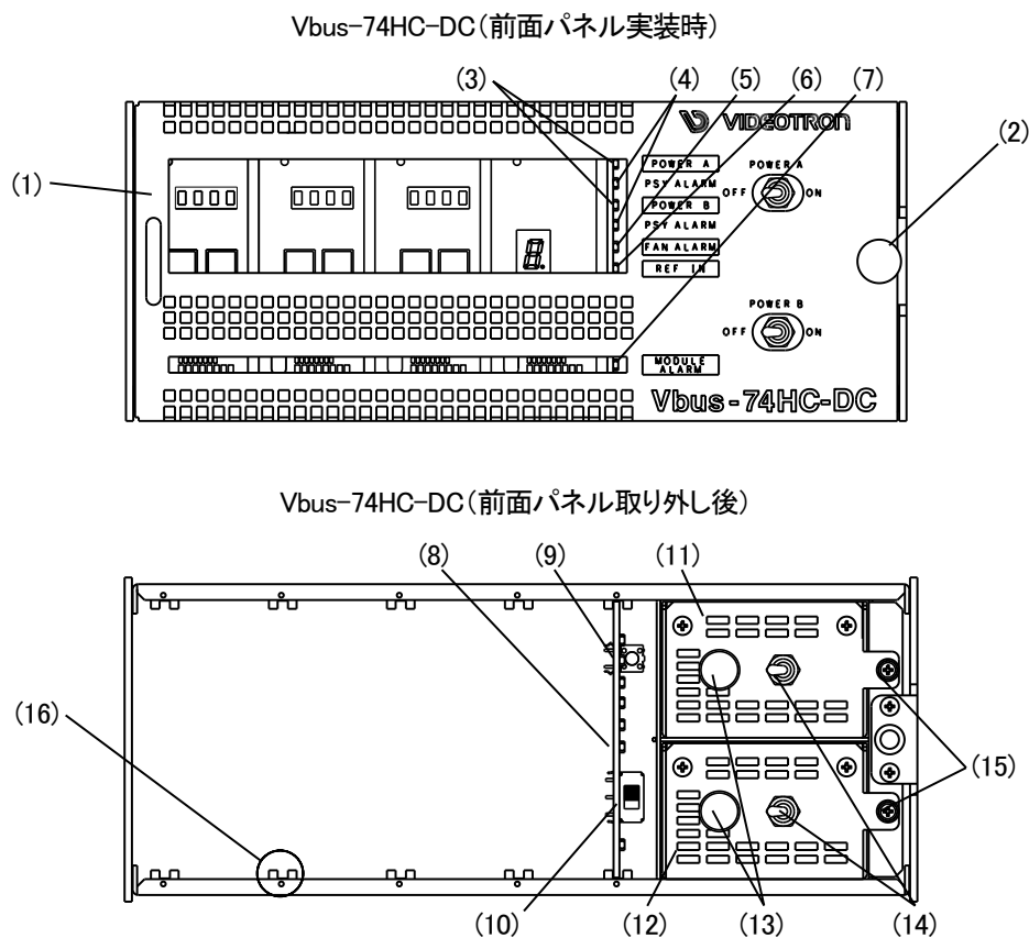
図 3-1 各部の名称(正面)
