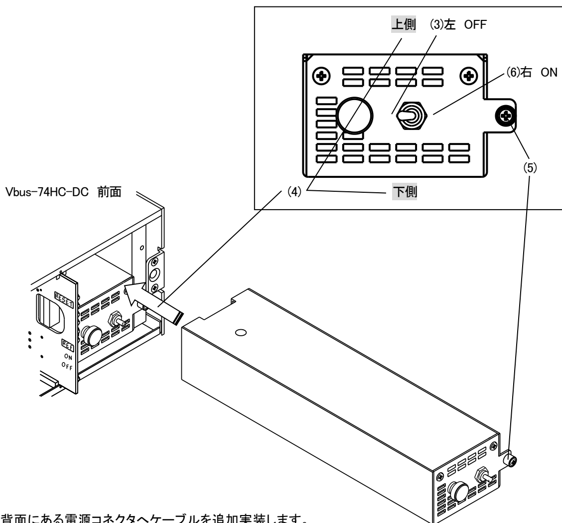
図 5-1 電源ユニット 増設方法
