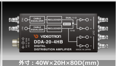
外寸: 40W×20H×80D(mm)
