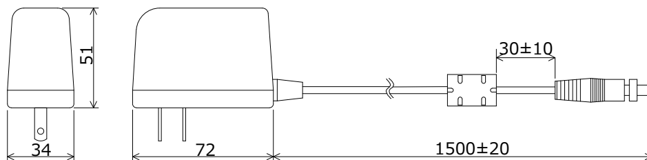
VAC-5V03AL(AC 電源アダプター)
