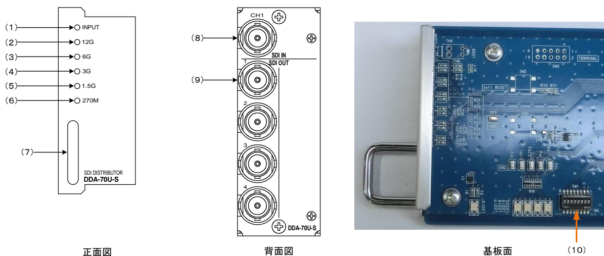
図 3.1 各部の名称
