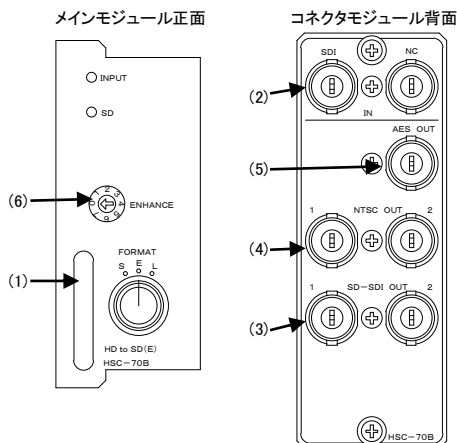
図4-1 操作方法
