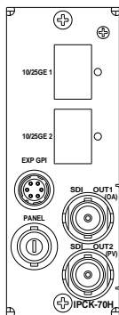
図2.1.2 コネクタモジュール背面図
