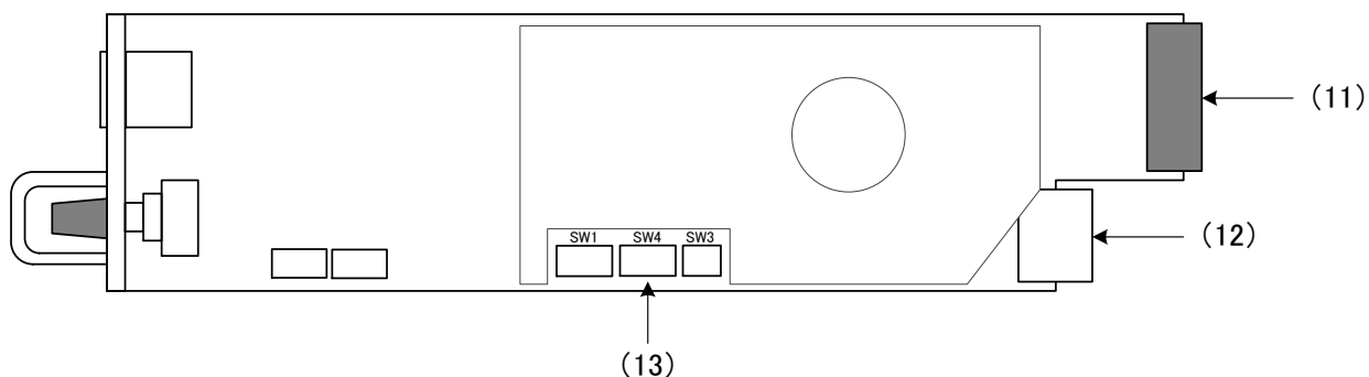
図 3.2 MTX-70-168HB モジュール基板面
