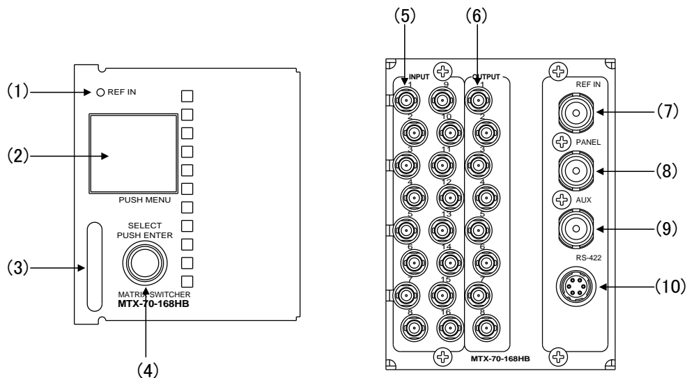
図 3.1 MTX-70-168HB モジュール/コネクタモジュール正面図
