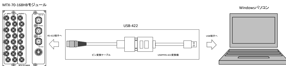
図 4.7a PC から RS-422 制御
