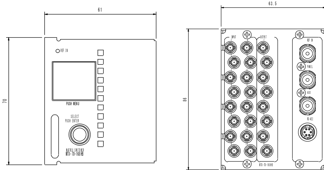
【MTX-70-168HB モジュール】
