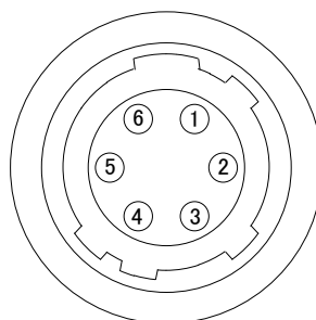
筐体背面から見たピン番号
