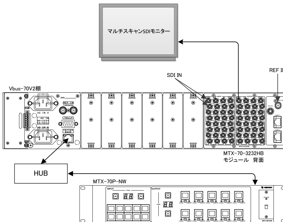
図 2.1 機能チェック接続図
