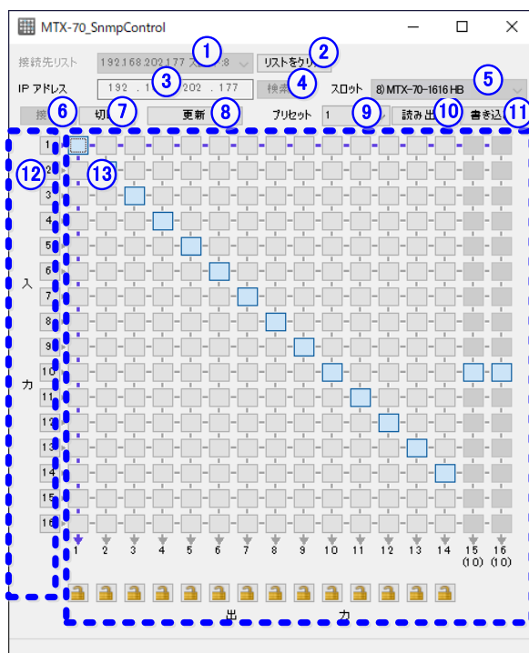
図 4.9 MTX-70 SNMP 制御画面説明
