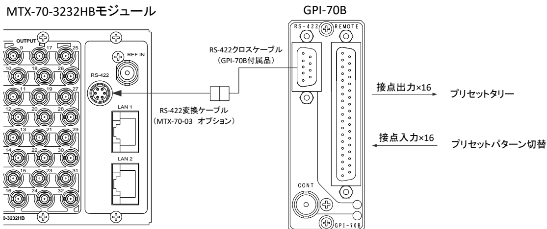
図 4.10 GPI-70B 接続図
