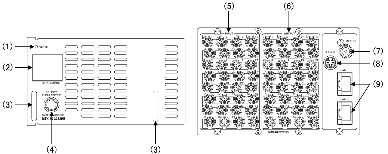
図 3.1 MTX-70-3232HB モジュール正面／背面
