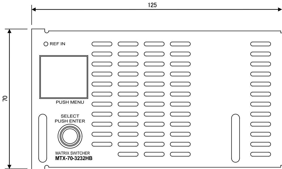
【MTX-70-3232HB モジュール】
