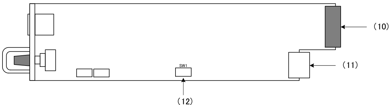
図 3.2 MTX-70-3232HB モジュール基板面図
