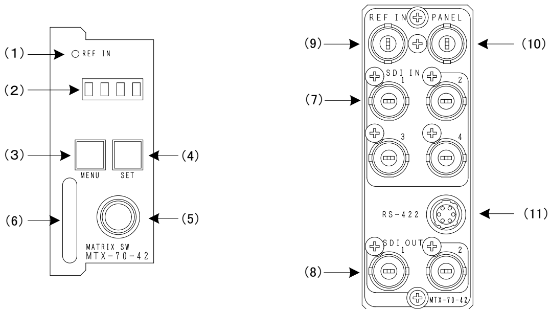
図 3.1 メインモジュール/コネクタモジュール正面図
