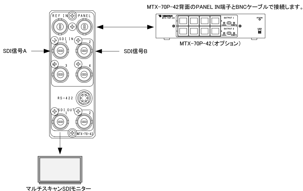
図 2.1 機能チェック接続図
