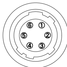
REMOTEコネクタ背面図 ヒロセ HR-10A-7R-6S (適合プラグ: HR-10A-7P-6P)
