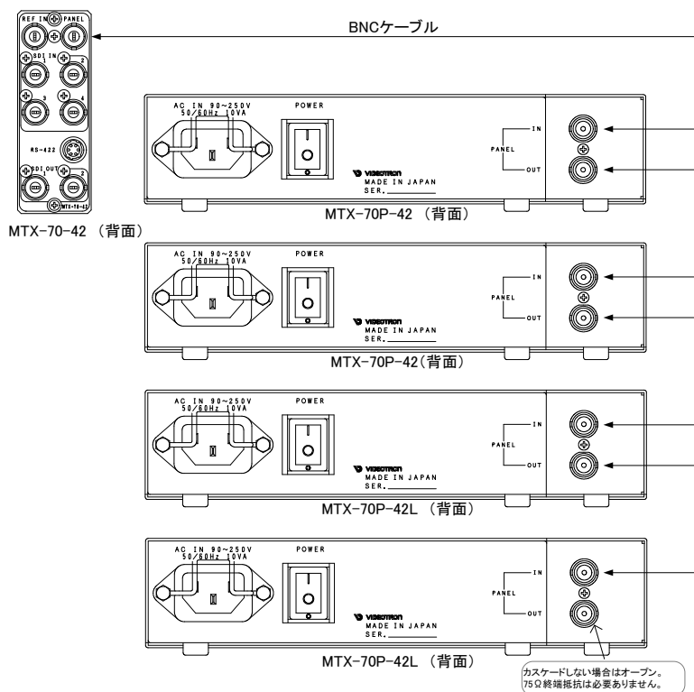
図4.122 カスケード接続例
