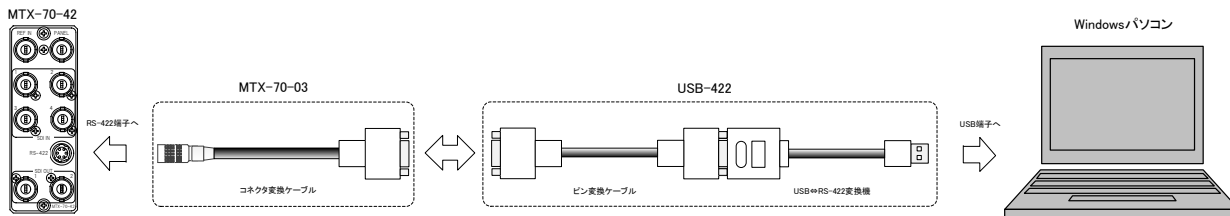
図 4.7a パソコンから RS-422 制御
