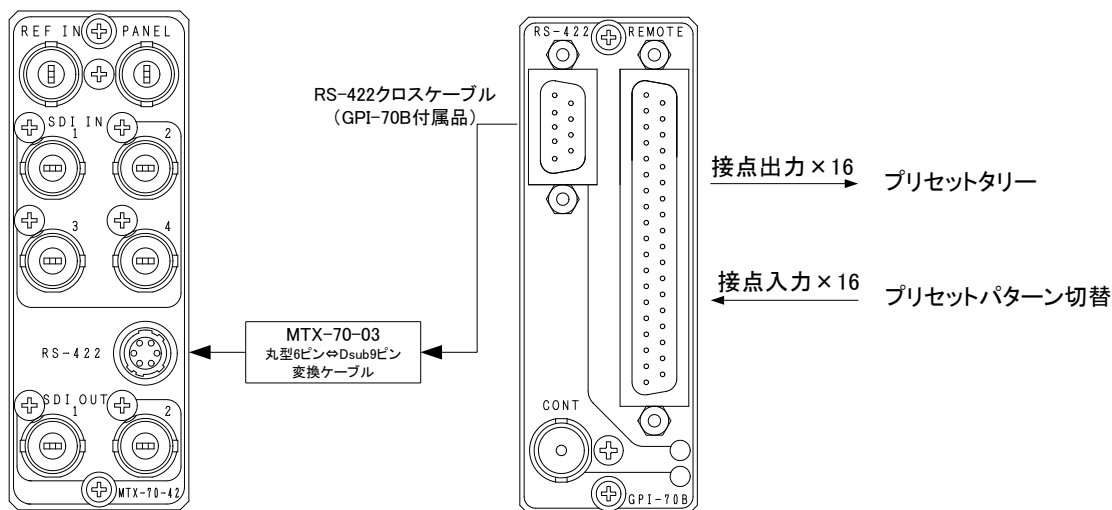
図 4.90 GPI-70B 接続図
