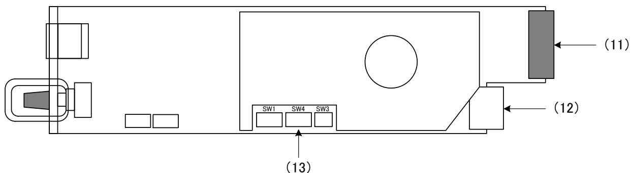
図 3.2 MTX-70-44HB モジュール基板面図
