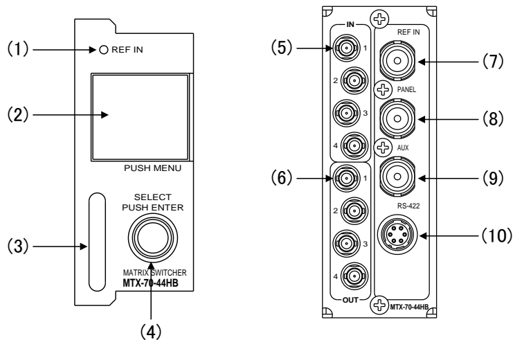
図 3.1 MTX-70-44HB モジュール/コネクタモジュール正面図
