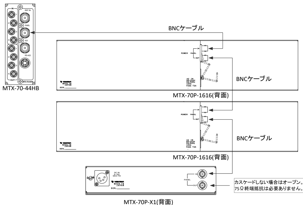
図4.122 カスケード接続例
