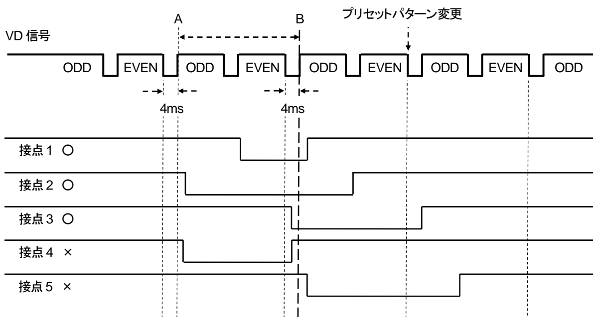
図 4.92 GPI-70B を使用した時のプリセットパターン切り換えタイミング
