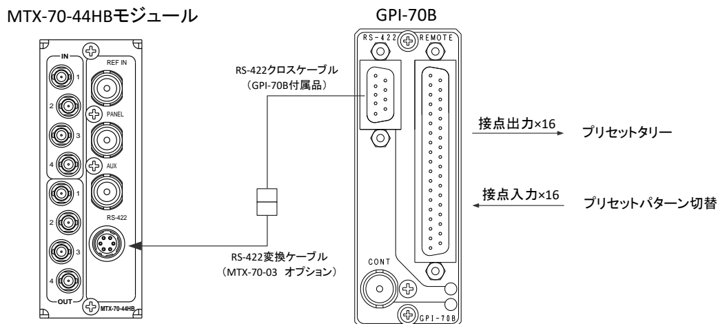
図 4.90 GPI-70B 接続図
