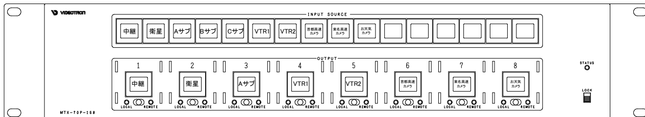
正面図
