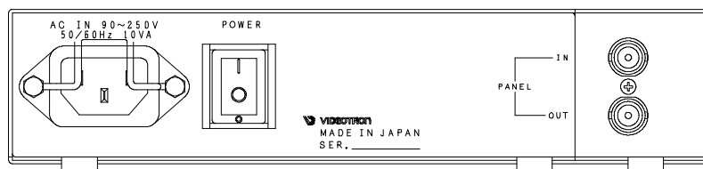
MTX-70P-42,L 背面図
