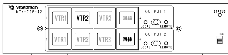
MTX-70P-42 正面図
