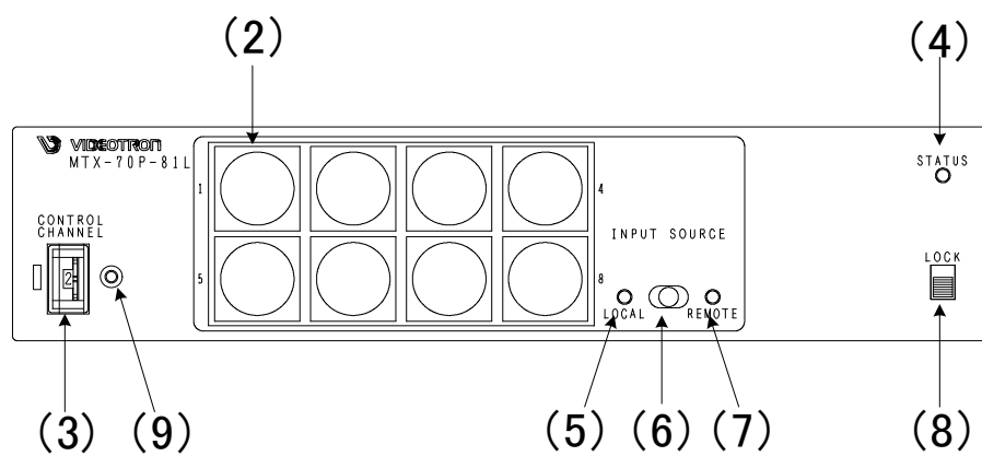
図 3.6 MTX-70P-81L 正面図
