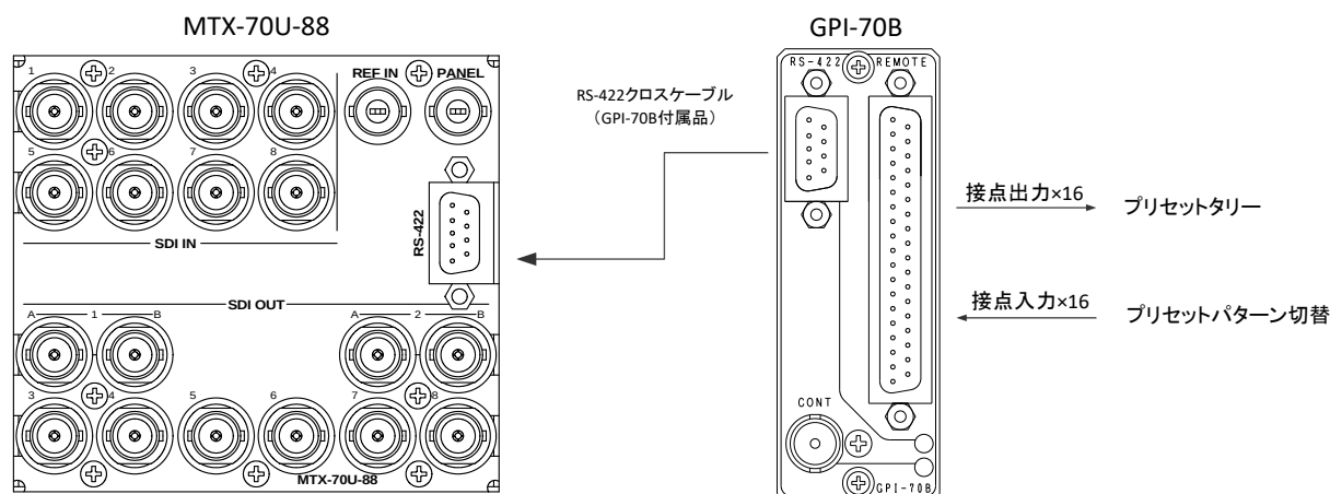
図 4.90 GPI-70B 接続図
