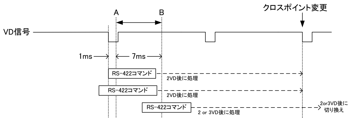
図 4.163 RS-422 制御タイミングチャート(DIPSW1=OFF)
