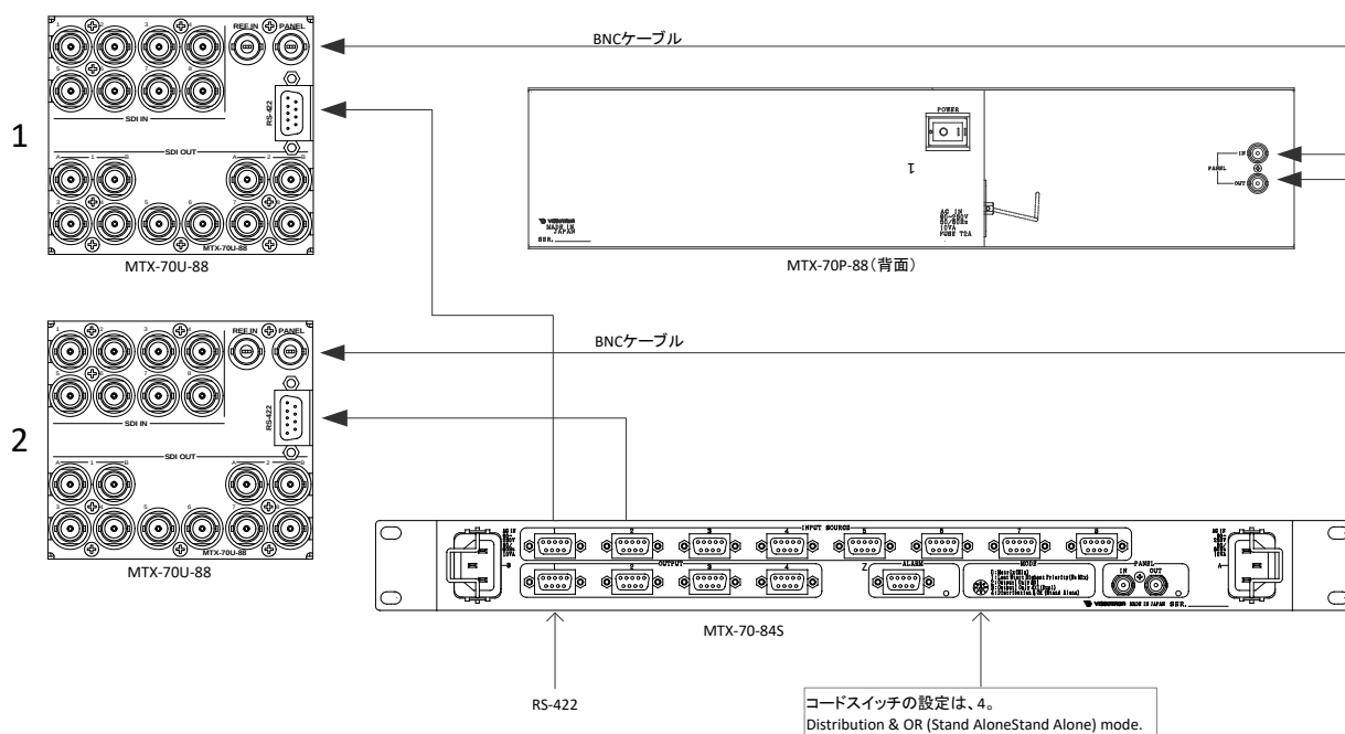
図4.161 パラレルモード接続図
