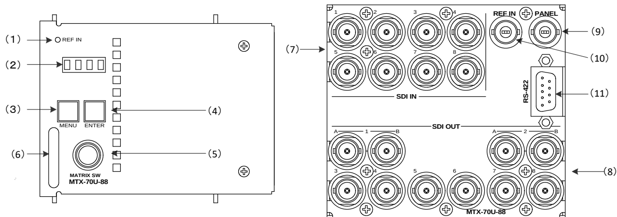
図 3.1 メインモジュール/コネクタモジュール正面図
