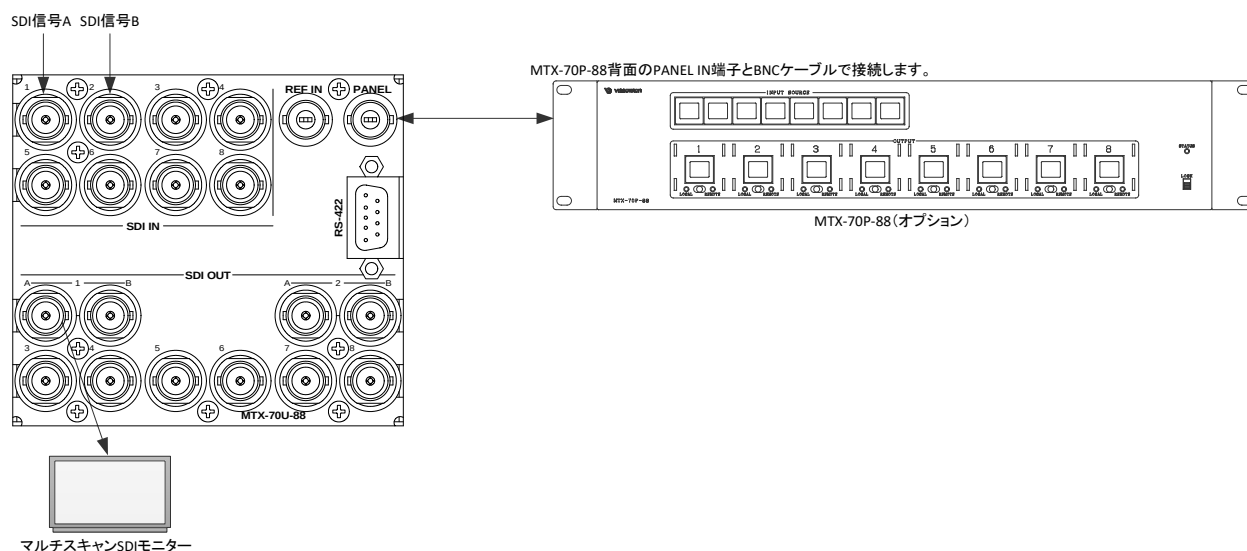
図 2.1 機能チェック接続図
