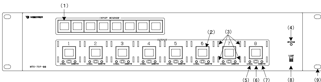
図 3.3 MTX-70P-88 正面図
