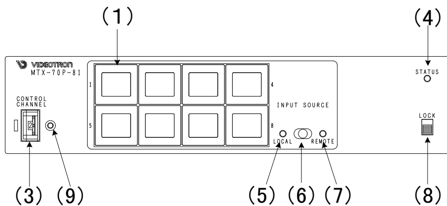
図 3.5 MTX-70P-81 正面図
