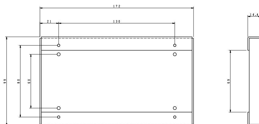
側板
